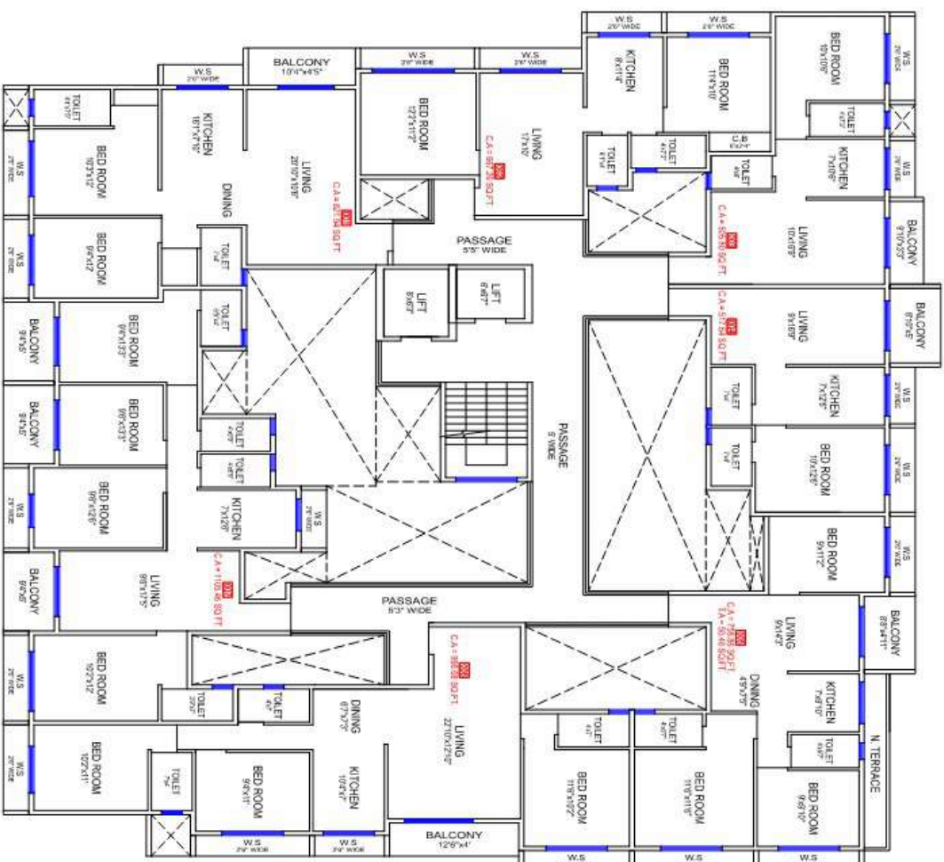
5TH FLOOR PLAN SCALE: N.T.S
