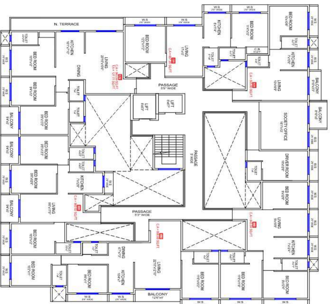
1ST FLOOR PLAN SCALE: N.T.S
